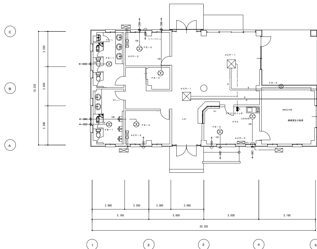
空調工事 S=1:100
