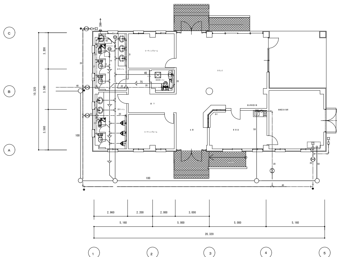
衛生工事 S=1:100
