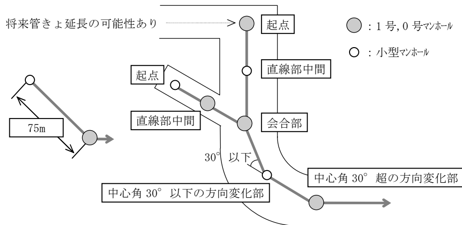
－小型マンホール設置基準モデル図－
