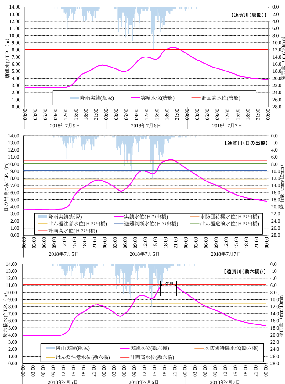
図 2.3.7(1) 河川水位（平成 30 (2018) 年 7 月 6 日）
