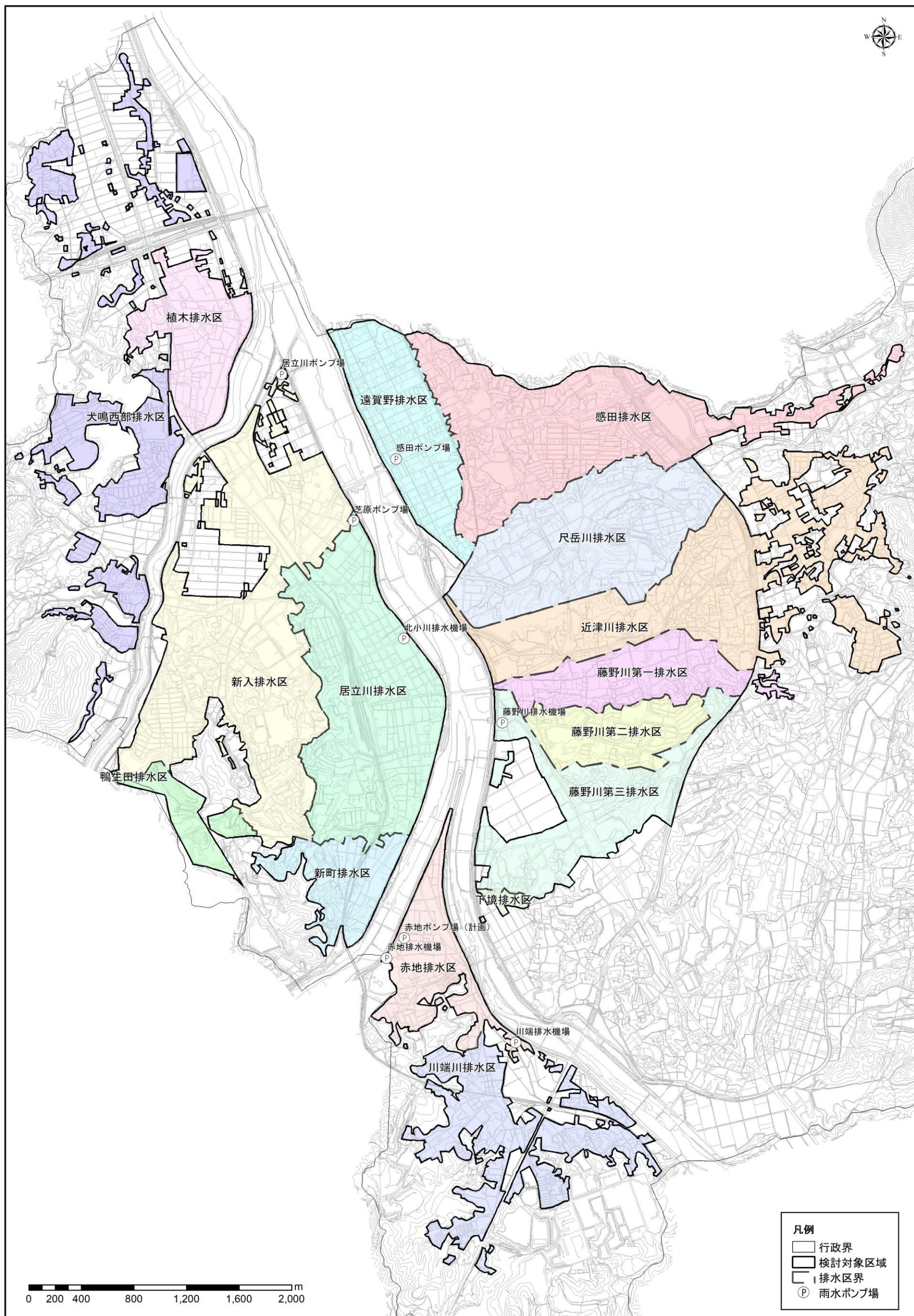
図 4.1.1 排水区の位置
