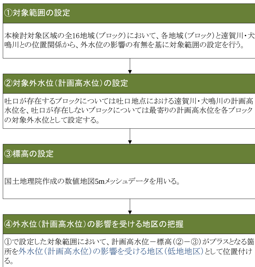
図 4.4.2 外水位（計画高水位）の影響把握フロー
