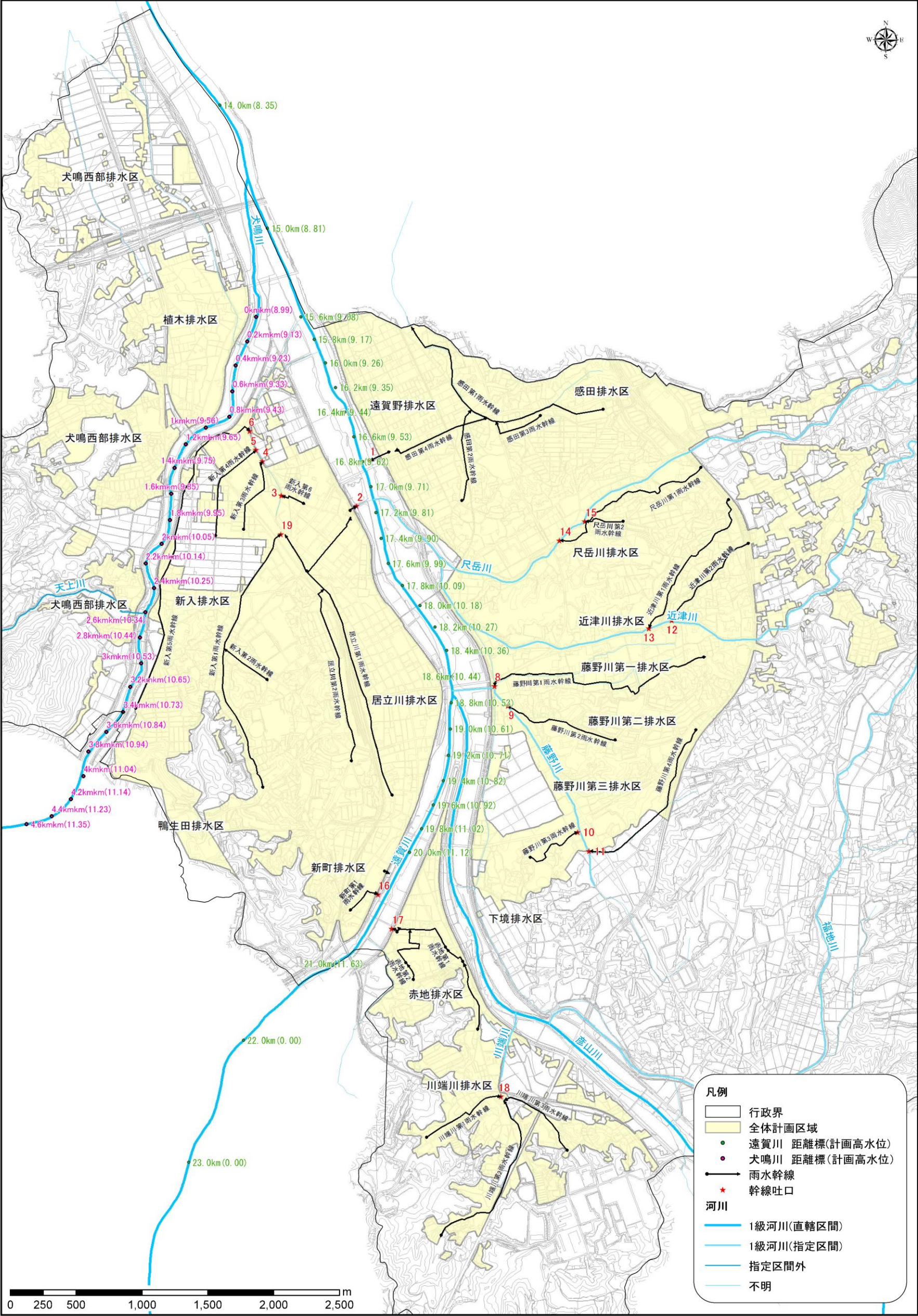
図 2.2.5 遠賀川・犬鳴川の計画高水位と吐口箇所の位置関係
