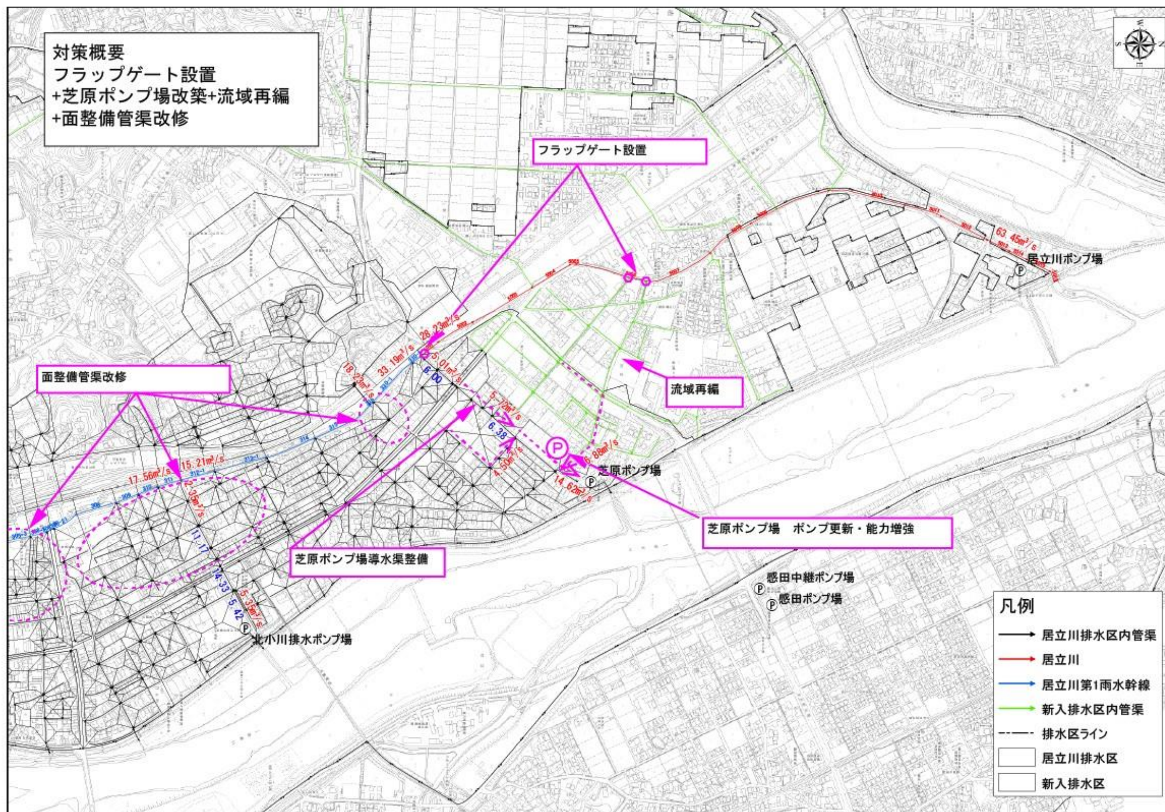
図 7.3.1 対策概要図
