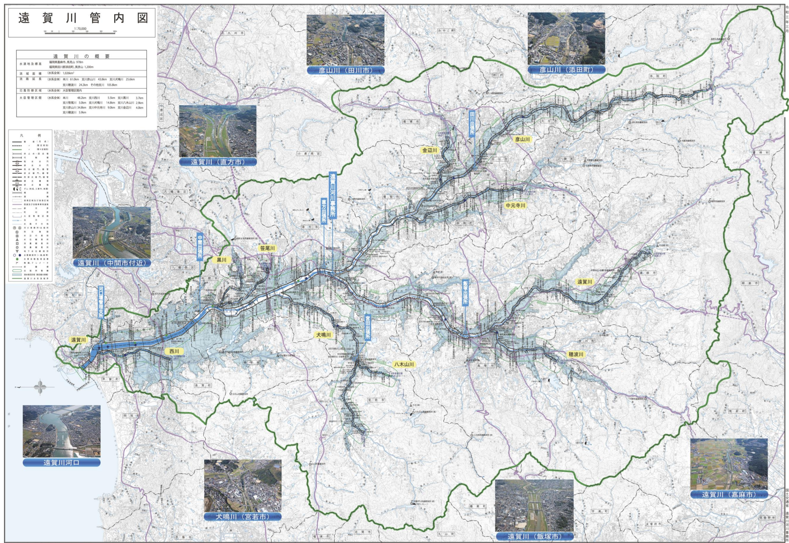
図 2.2.4 遠賀川管内図【直轄区間】[収集資料⑨]
