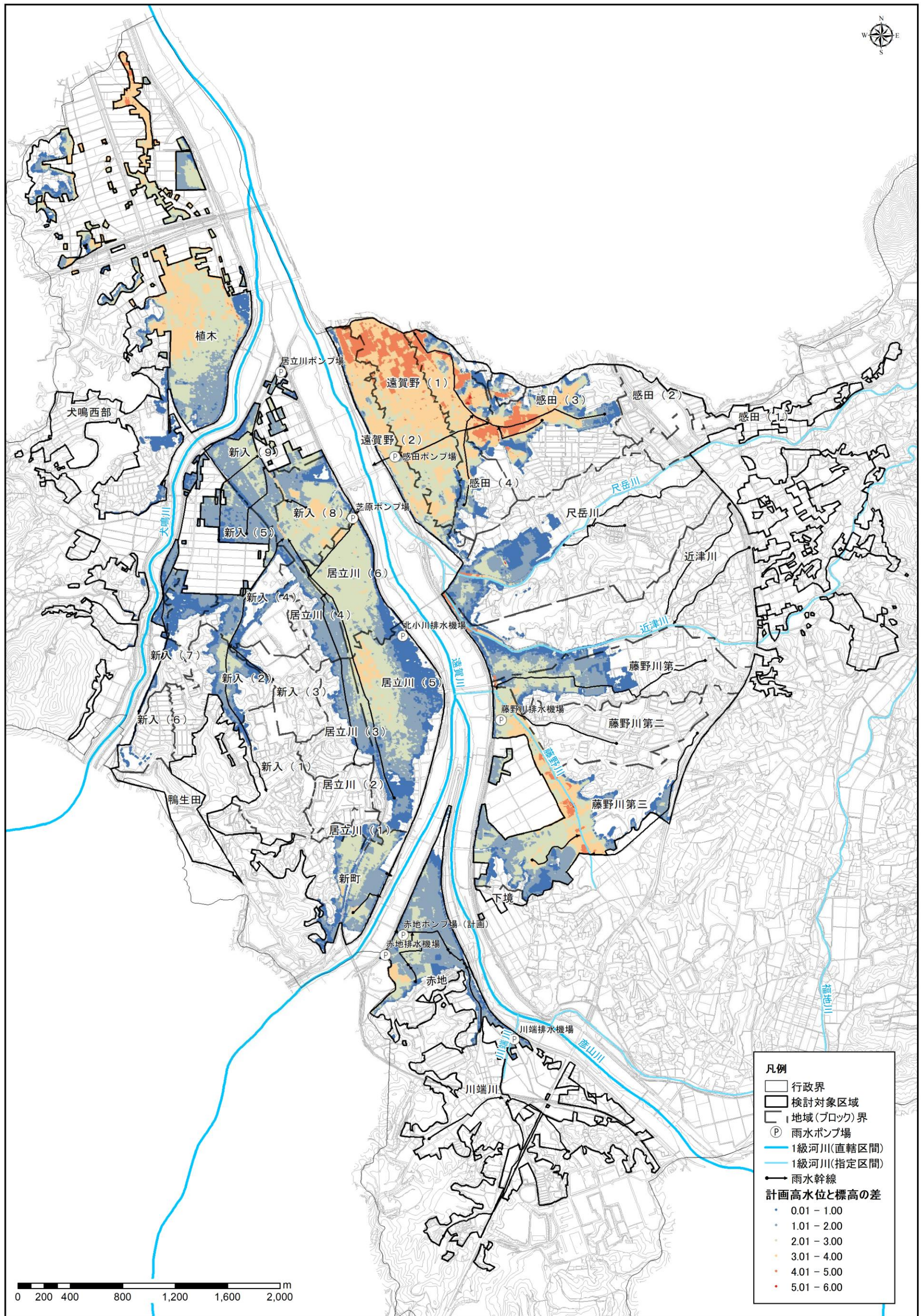
図 4.4.5 外水位（計画高水位）による影響評価図（計画高水位－5m標高）
