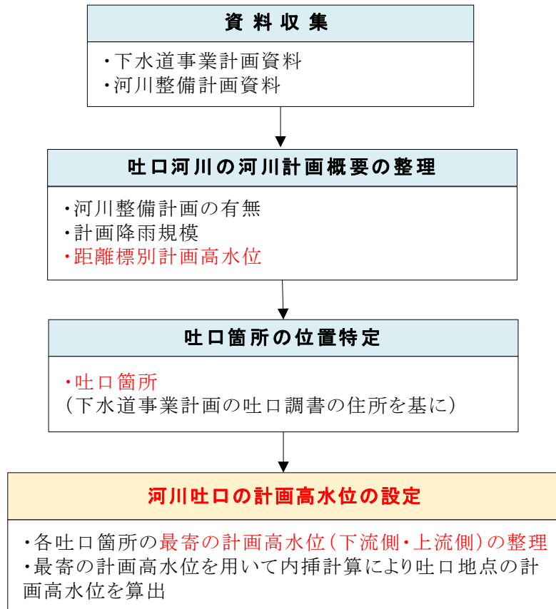
図 2.2.2 河川吐口の計画高水位の設定フロー
