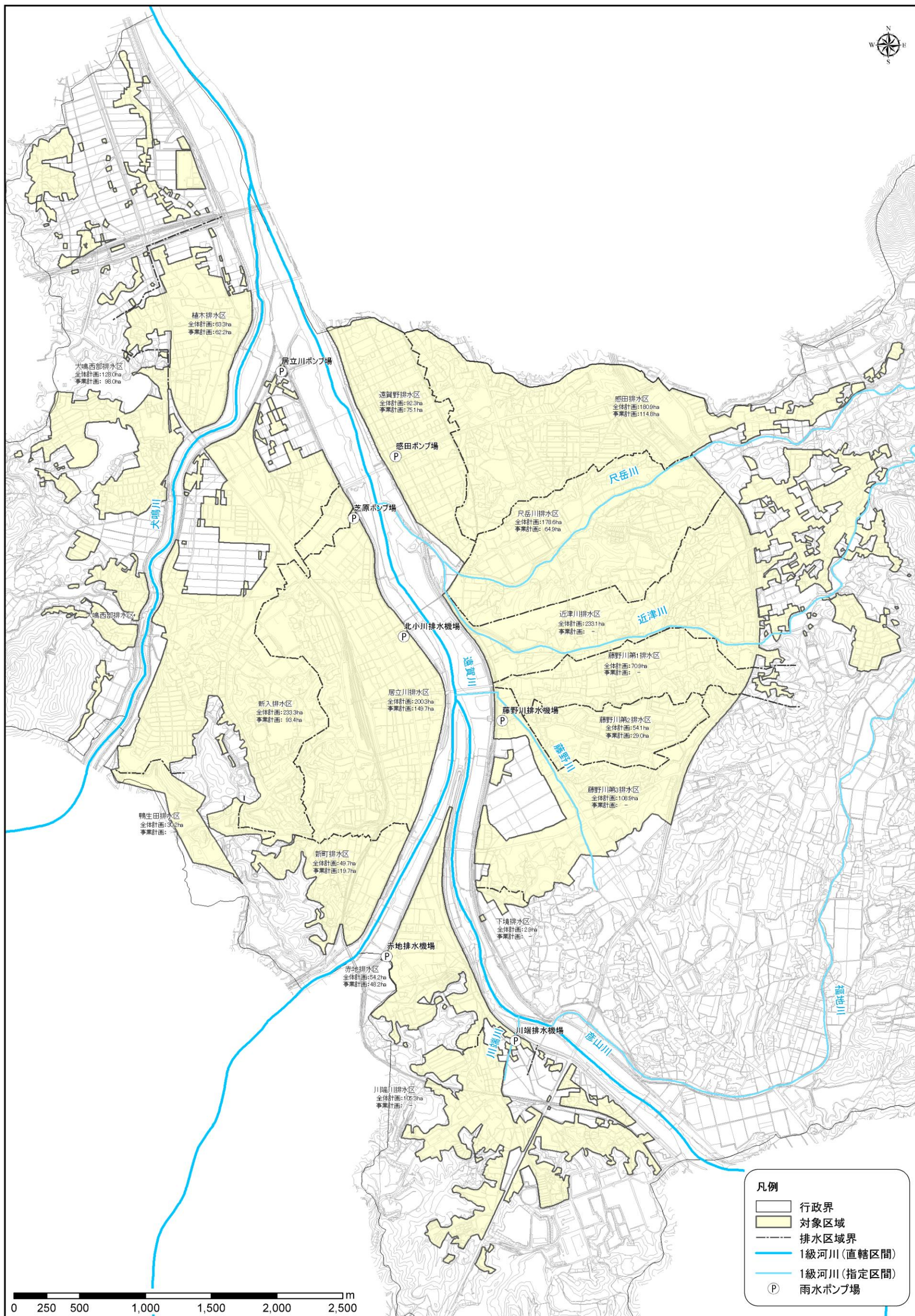
図 2.1.1 排水区及び雨水ポンプ場位置図
