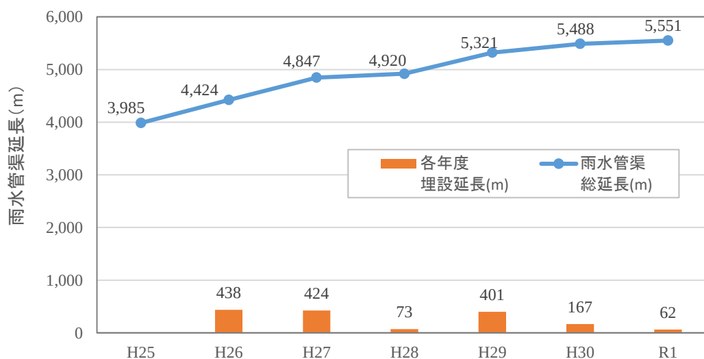
図 2.4.1 年度別雨水管渠延長の推移
