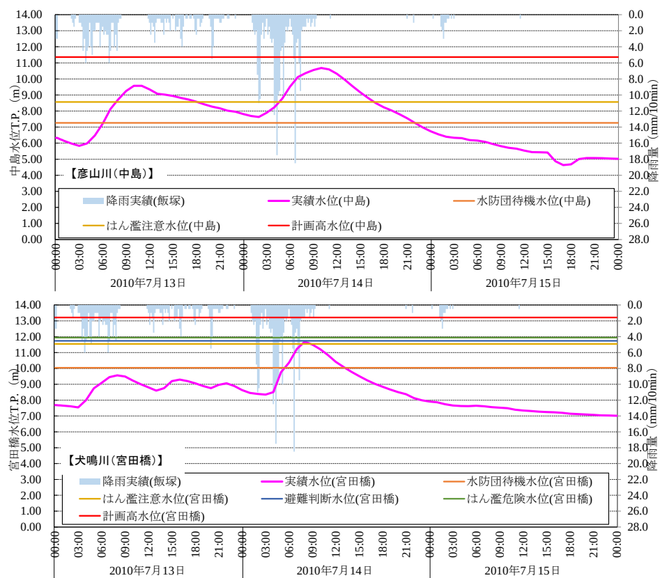
図 2.3.5(2) 河川水位 (平成 22 (2010) 年 7 月 14 日)
