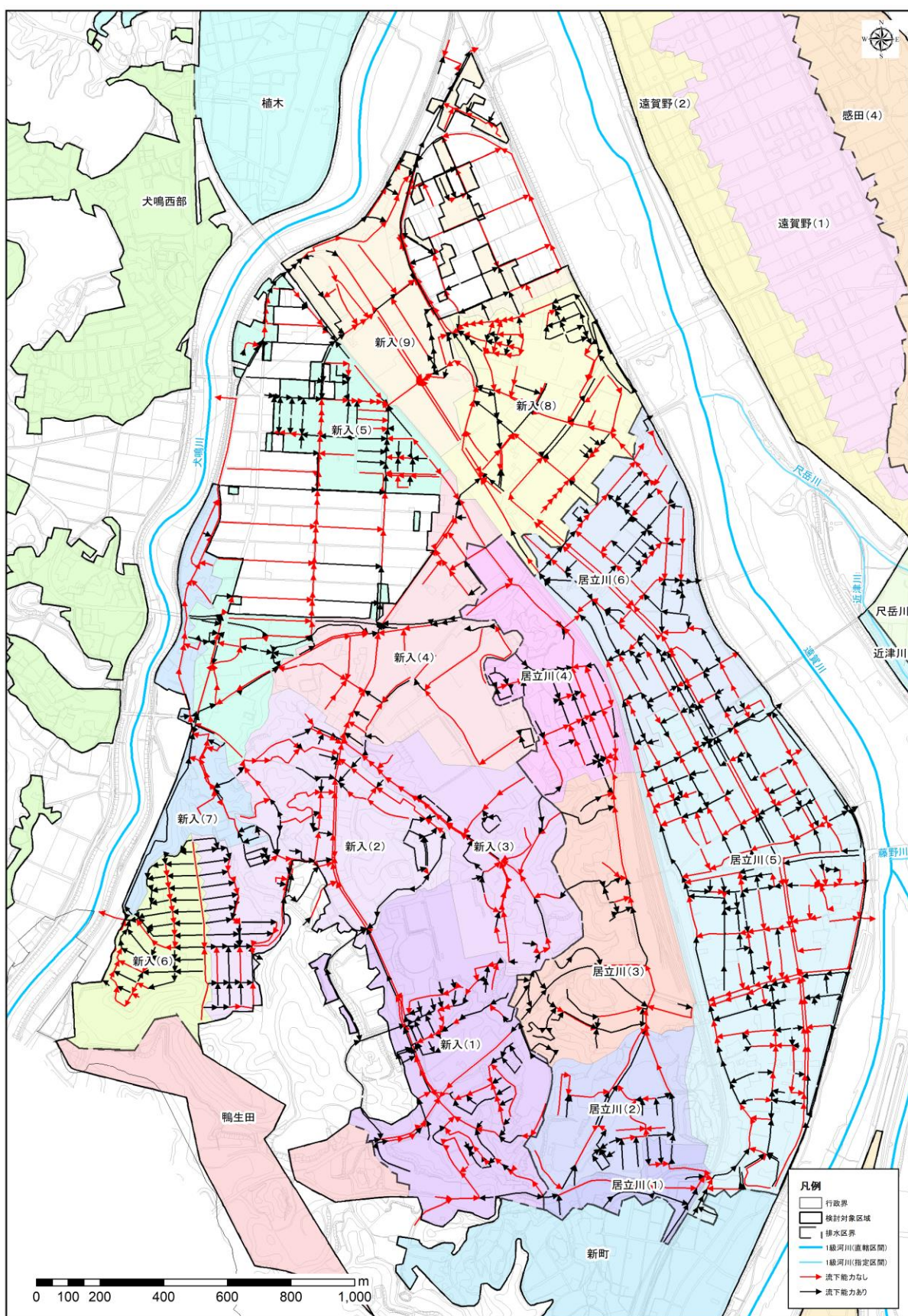
図 4.4.12 新入・居立川排水区における雨水管渠の能力評価結果
