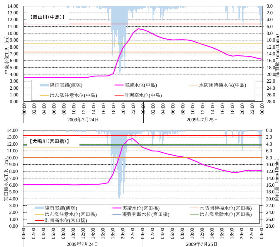
図 2.3.4(2) 河川水位 (平成 21 (2009) 年 7 月 24 日)
