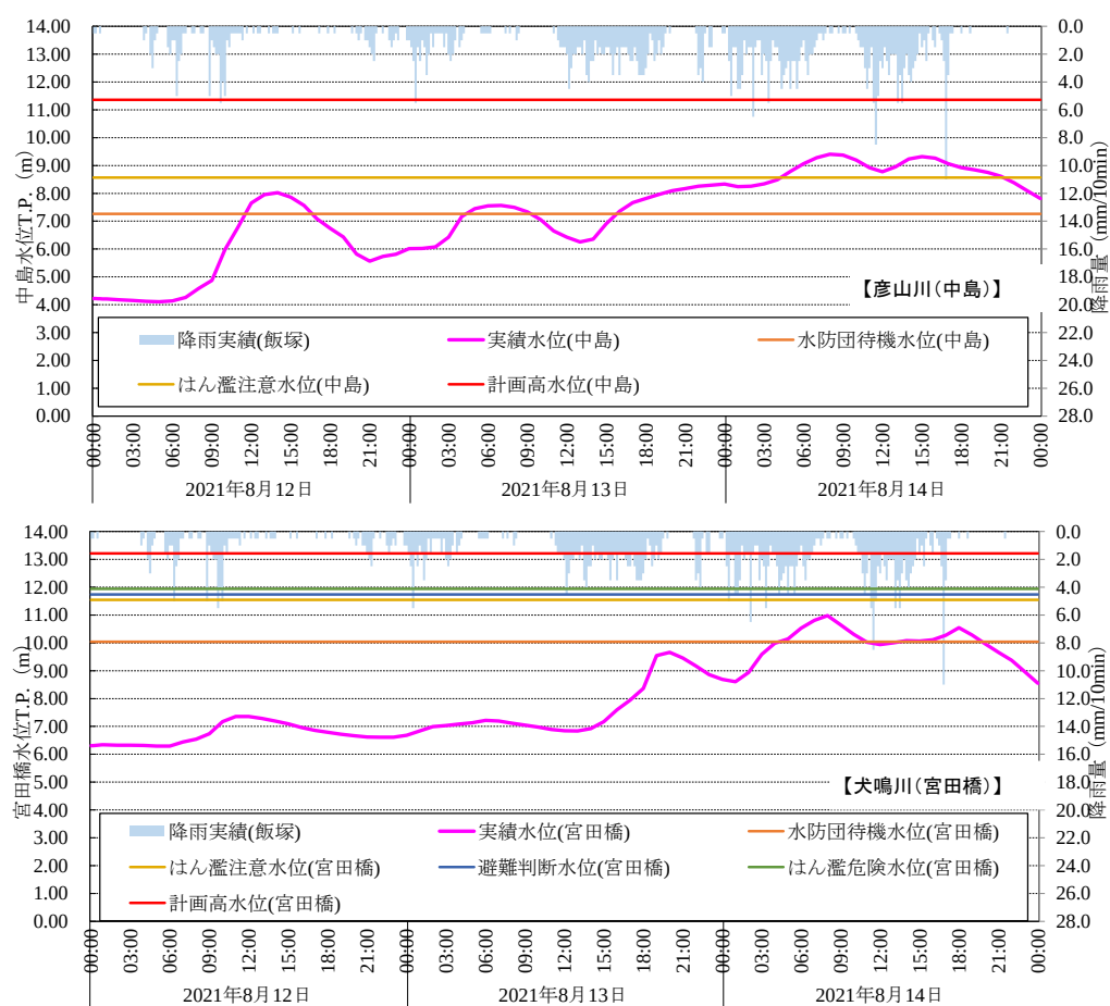
図 2.3.8(2) 河川水位 (令和3(2021)年8月14日)
