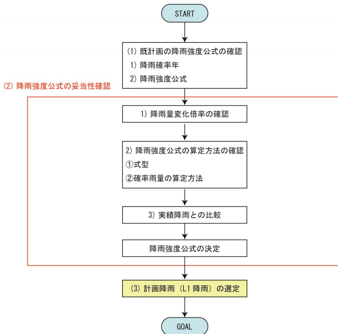
図 5.3.1 計画降雨（L1 降雨）選定フロー
