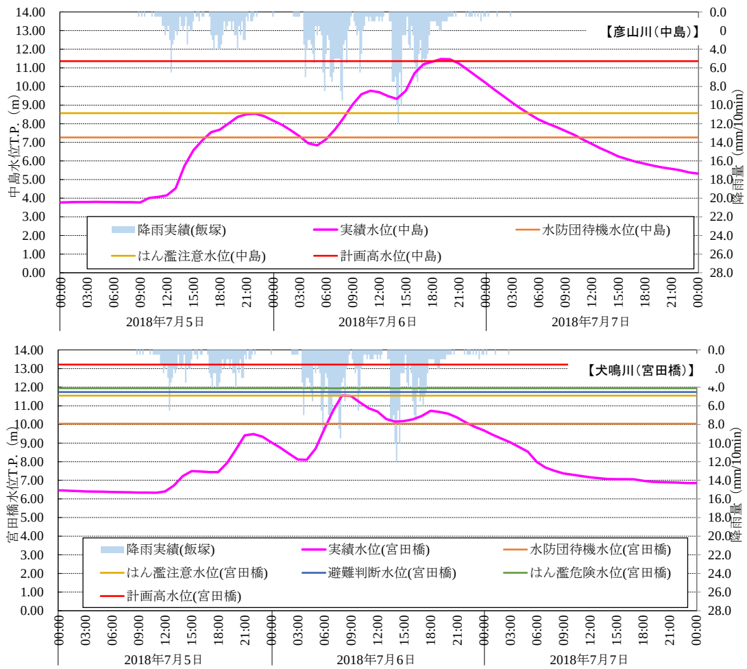
図 2.3.7(2) 河川水位 (平成 30 (2018) 年 7 月 6 日)
