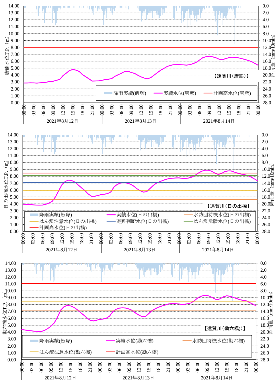
図 2.3.8(1) 河川水位（令和3(2021)年8月14日）
