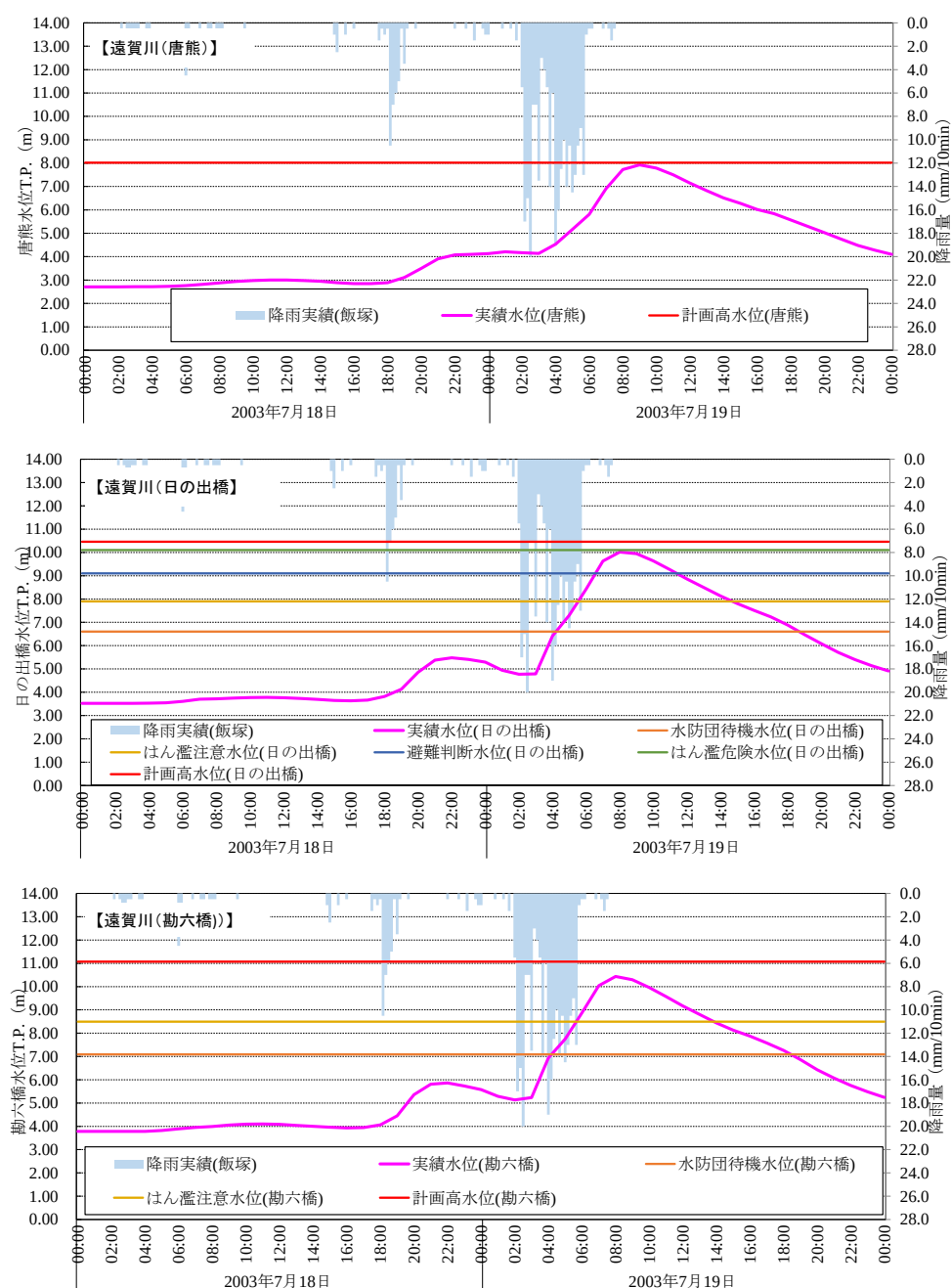
図 2.3.3(1) 河川水位（平成 15 (2003) 年 7 月 18 日）
