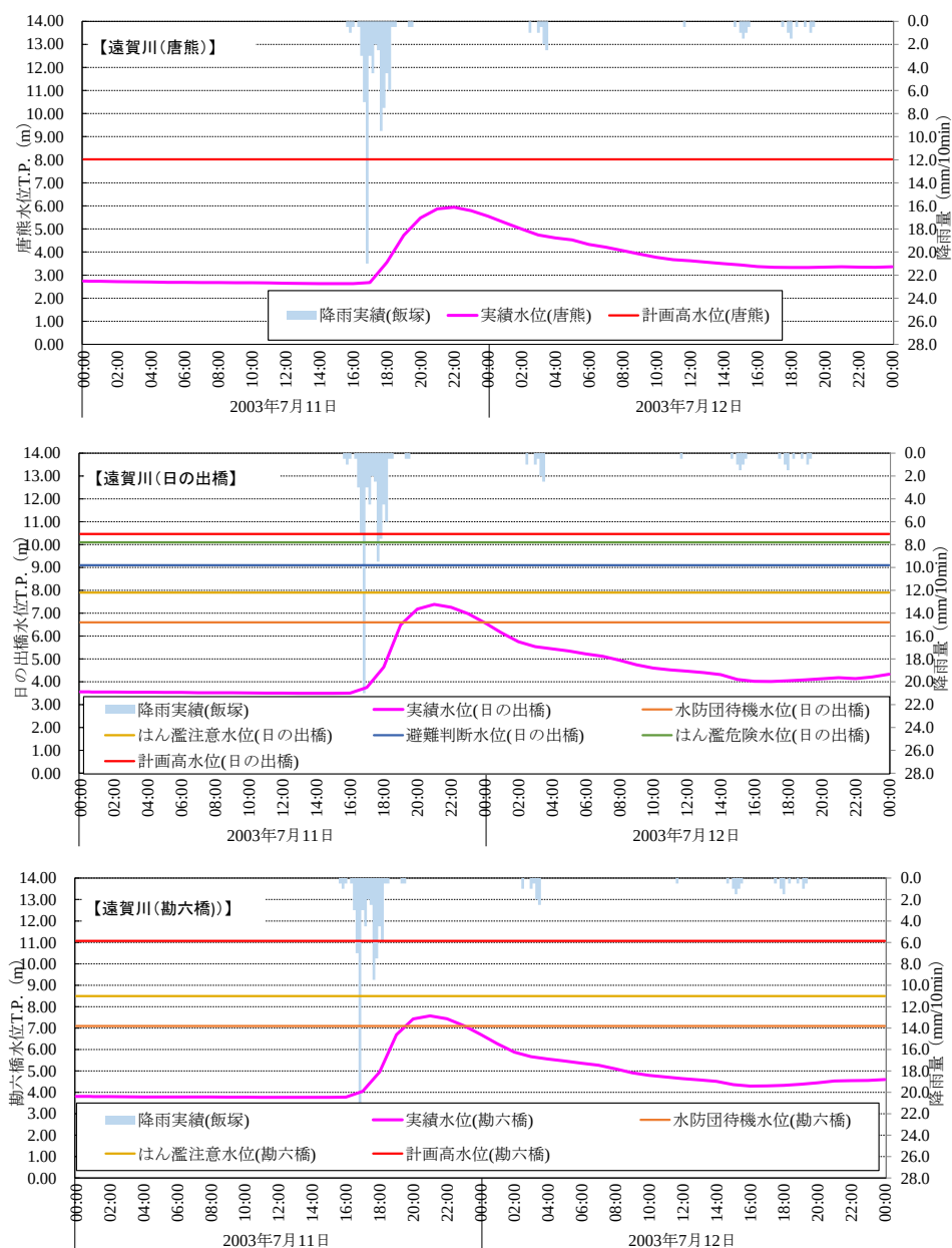
図 2.3.2(1) 河川水位 (平成 15 (2003) 年 7 月 11 日)
