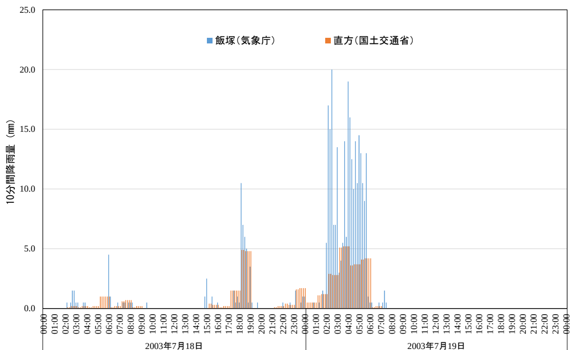
図 2.2.3 10 分雨量の時系列変化 (平成 15 (2003) 年 7 月 18 日降雨)
