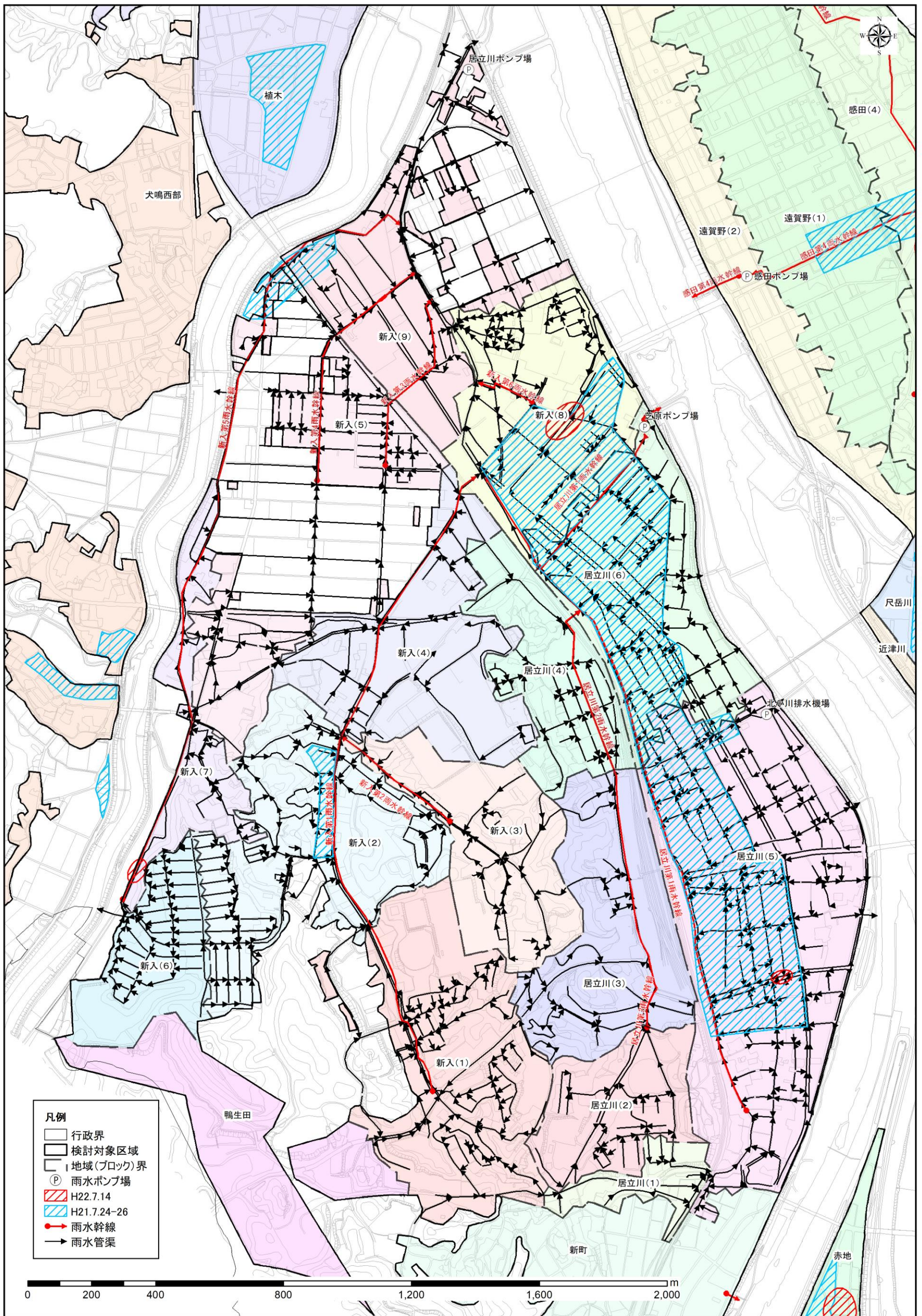
図 4.2.3 新入・居立川排水区のブロック分割に用いた管渠及び幹線の位置
