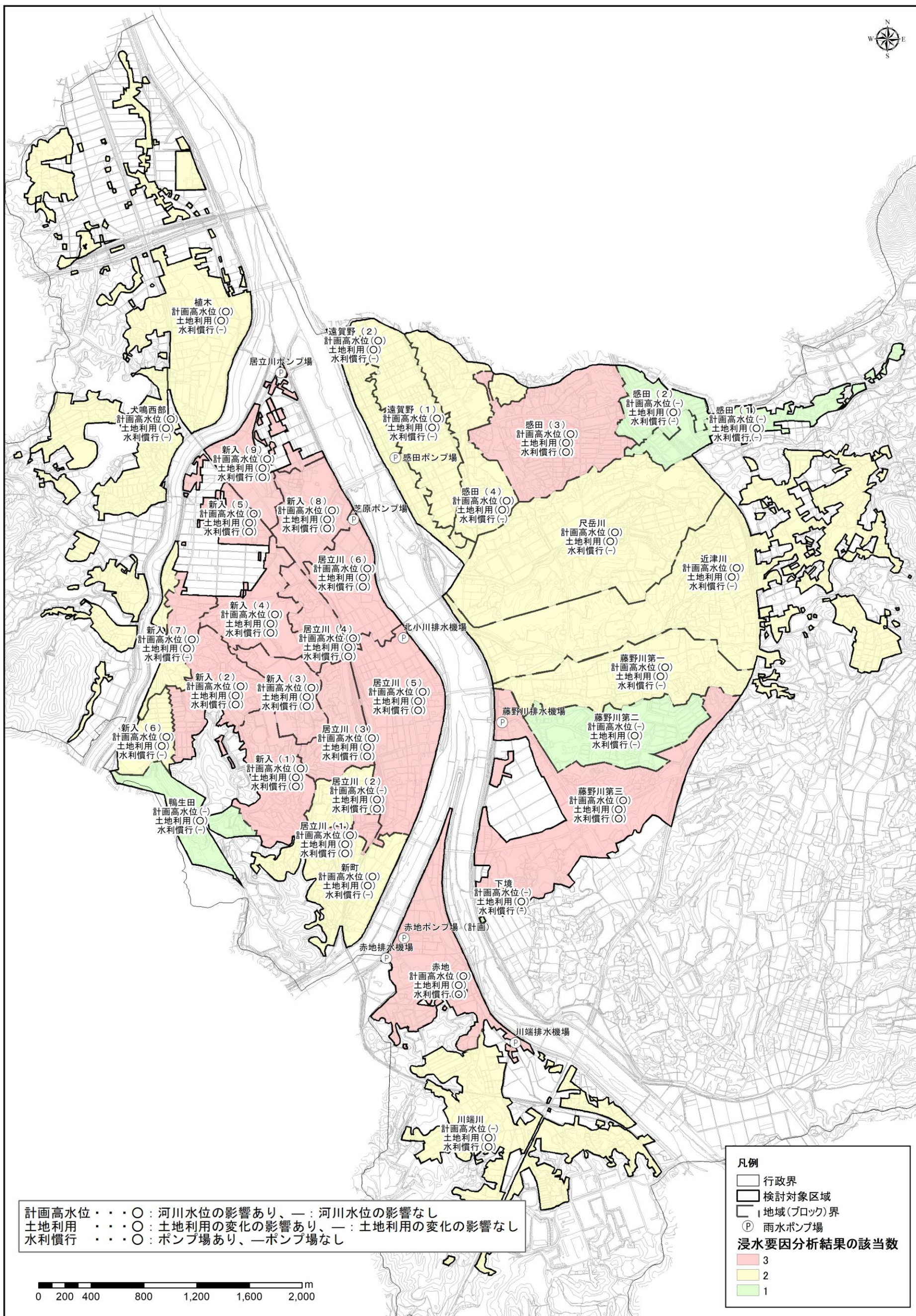
図 4.4.15 浸水要因分析結果（河川と水路の要因を除く）
