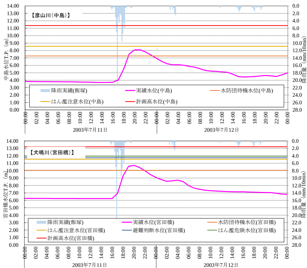
図 2.3.2(2) 河川水位 (平成 15 (2003) 年 7 月 11 日)
