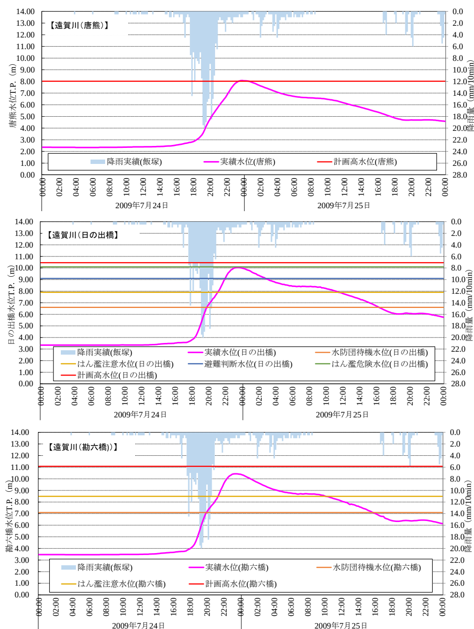
図 2.3.4(1) 河川水位（平成 21 (2009) 年 7 月 24 日）
