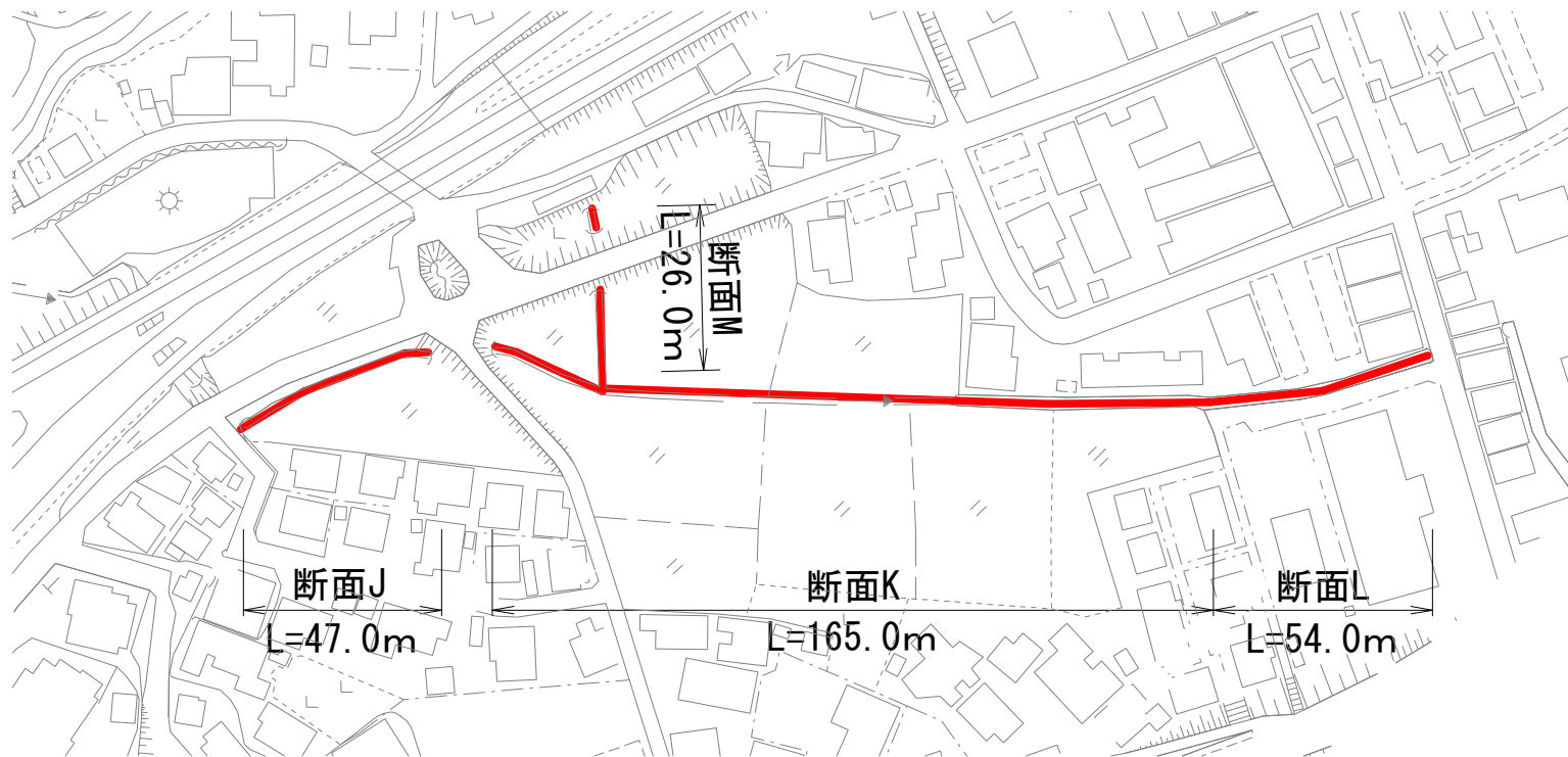
断面J L=47.0m
