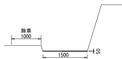
断面C L=25.0m
