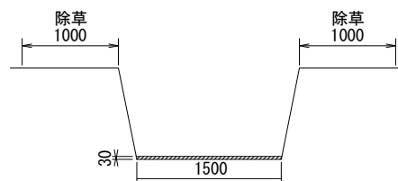
断面K L=165.0m
