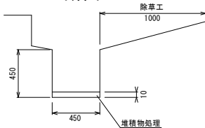
B断面
