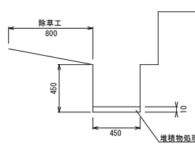
E断面
