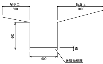
A断面
