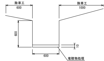
F断面
