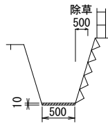
断面B L=19.0m
