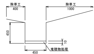
C断面
