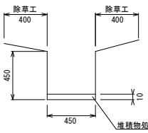
D断面
