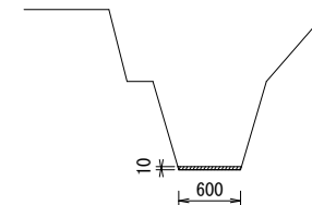
断面G L=38.0m
