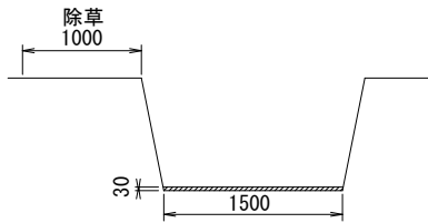
断面J L=47.0m
