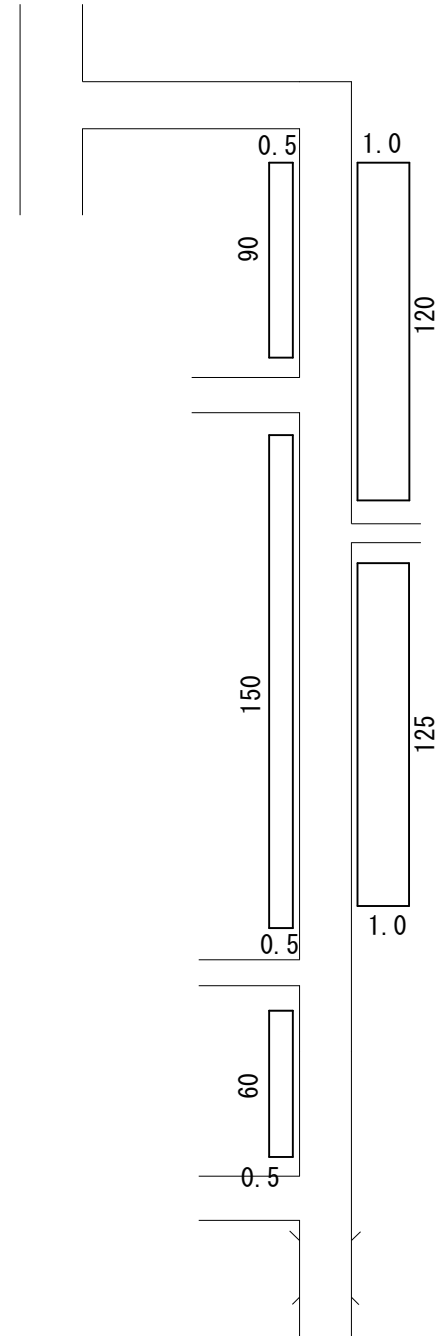
展開図(3工区)
