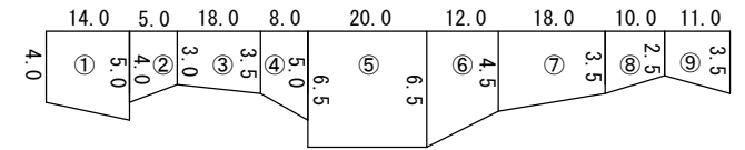
法面1 展開図
